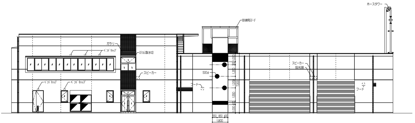
北立面図
