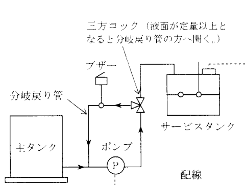
第4-1図 分岐装置
