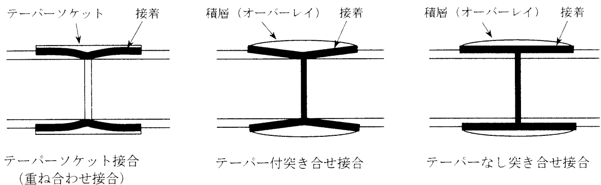
第4－5図 FRP配管の接着接合例
