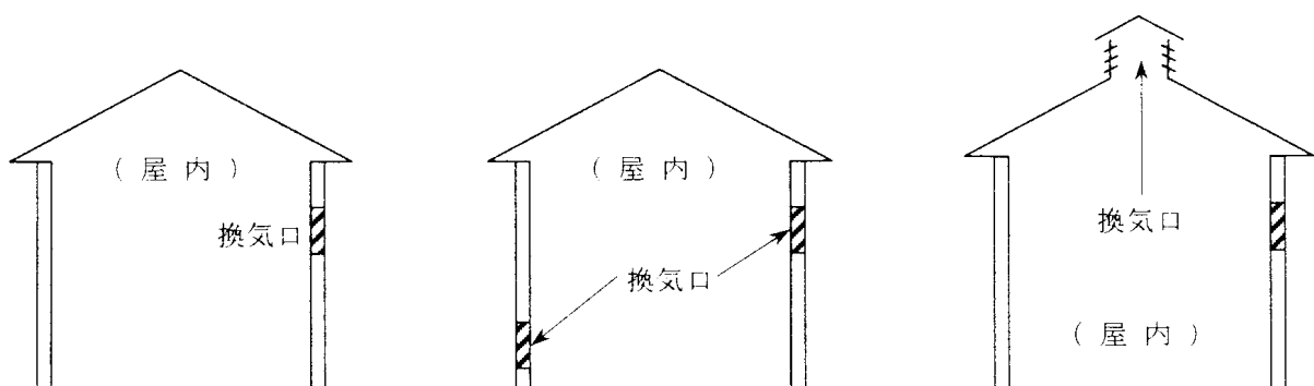
第4－19図 自然換気設備の例
