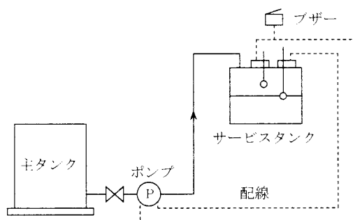
第4-3図 二重フロートスイッチによるポンプ停止装置
