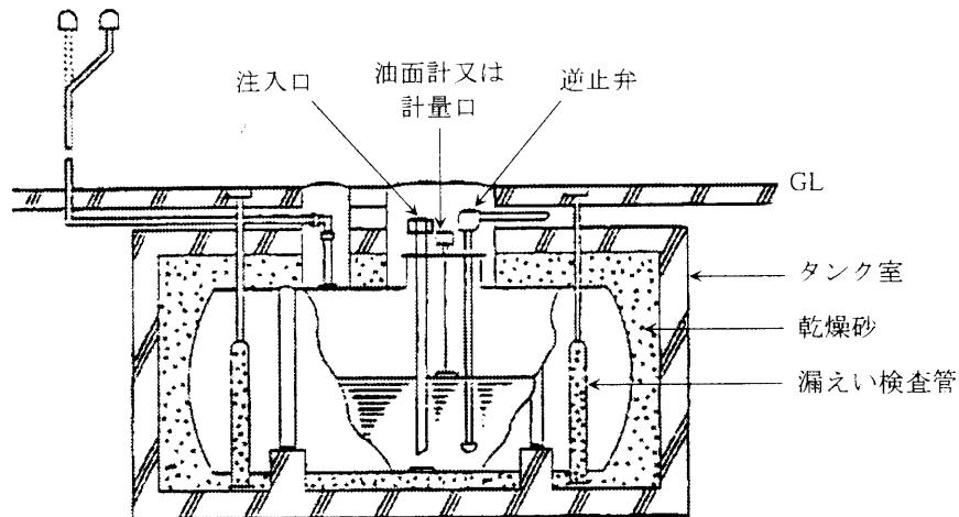
第4-35図 タンク室に設置する例
