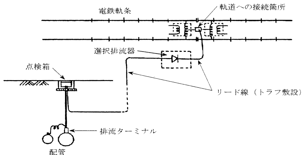
第4-11図 選択排流方式の例
