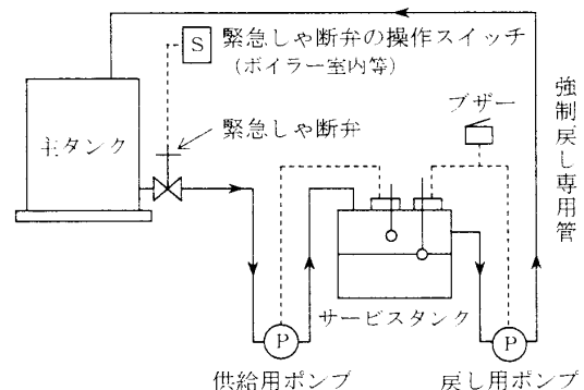
第4-4図 強制戻し専用管及び緊急しや断弁
