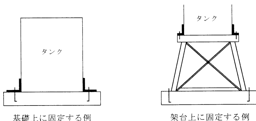
第4-30図 タンクの固定例
