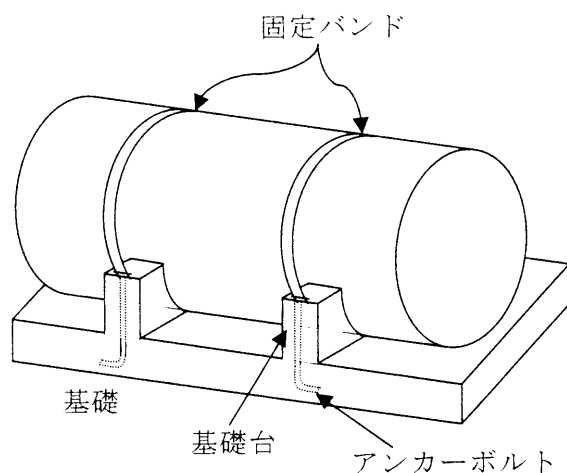
第4-31図 円筒横置型タンクの設置例
