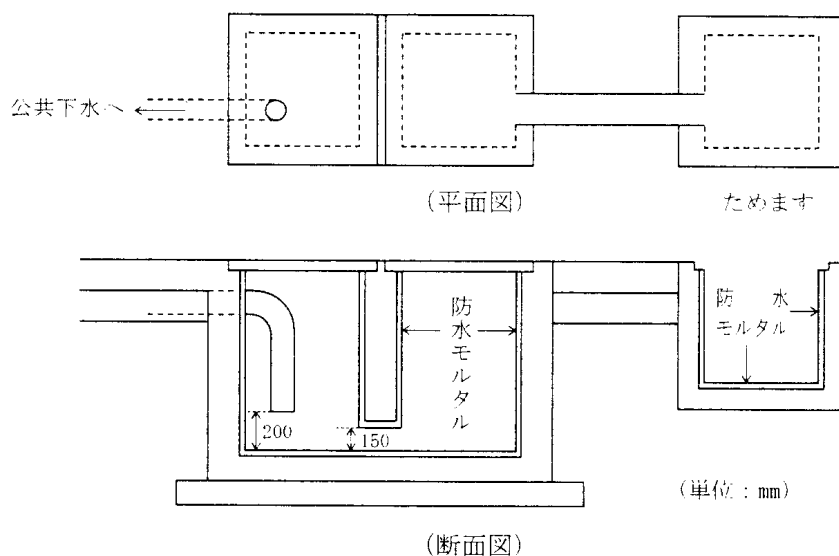
第４－１６図 ためます及び油分離槽の例
