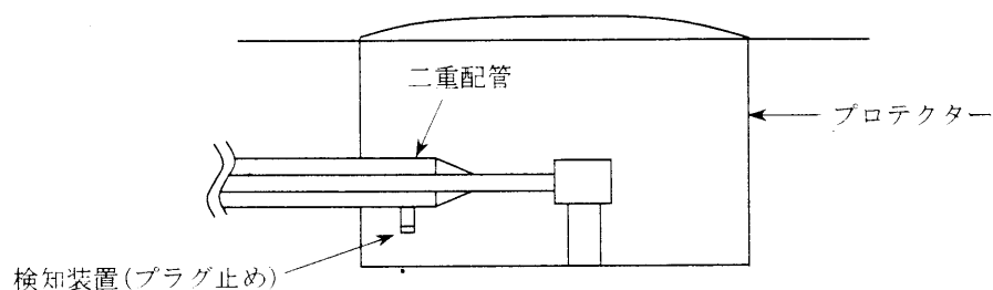
第4-12図 地下埋設配管を二重配管とし、検知装置を設ける方法
