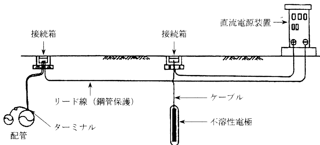
第４－１０図 外部電源方式の例
