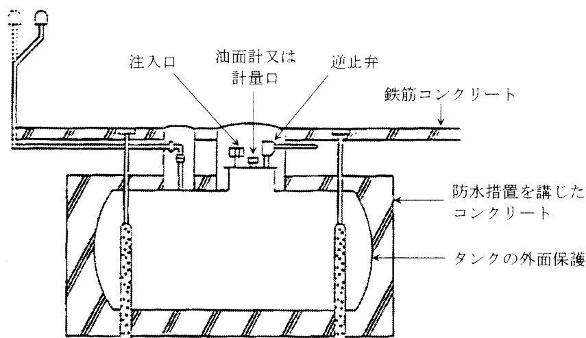
第4-36図 漏れ防止構造を有するタンクを設置する例
