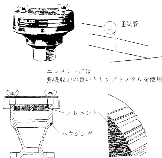
第8-1図 クリンプトメタル方式の引火防止装置の構造例
