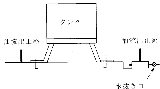
第6-2図 雨覆いを設けない例
