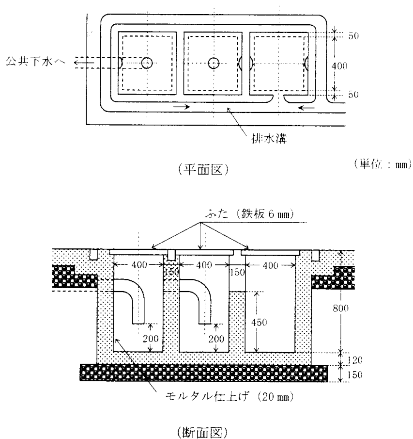
第４－１７図 油分離槽の例
