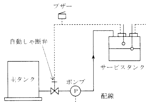
第4-2図 二重フロートスイッチによるしや断弁
