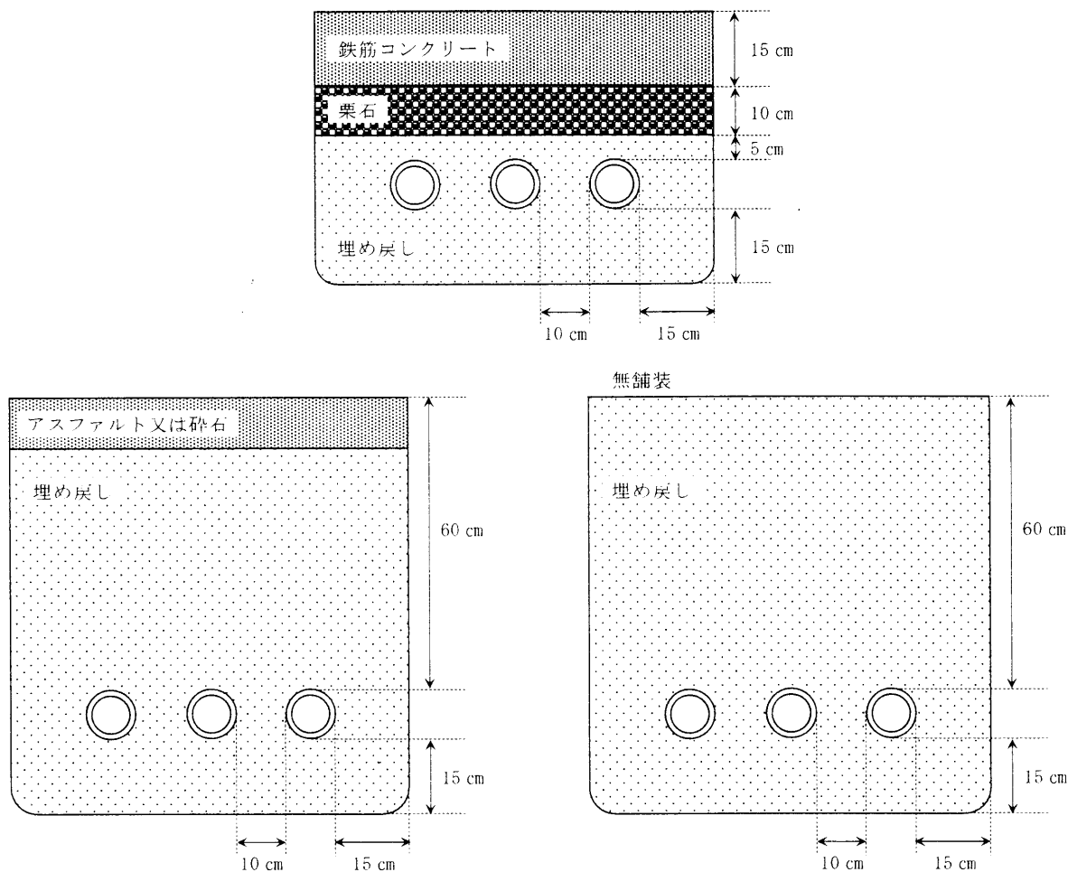
第4－8図 配管の埋設構造例
