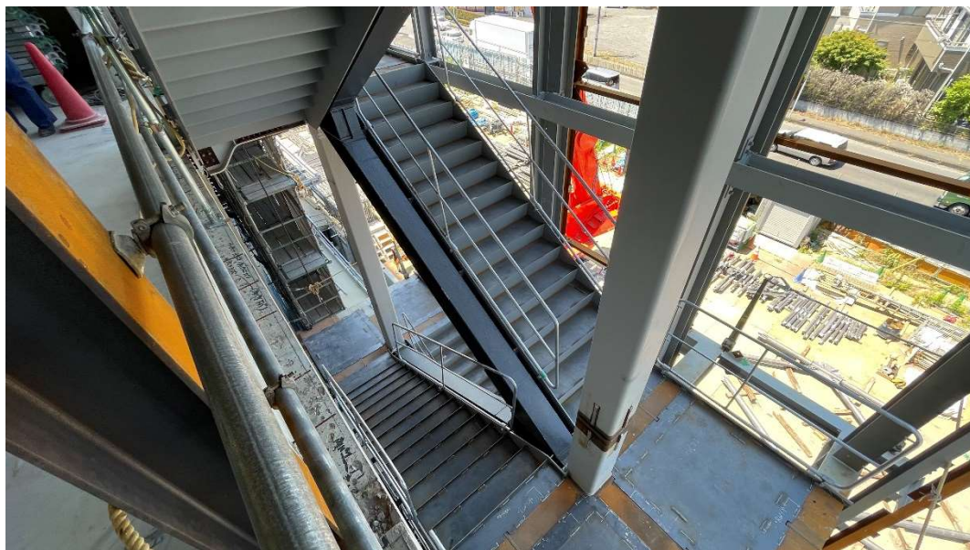
西側鉄骨階段工事状況 [2025.7月下旬]
