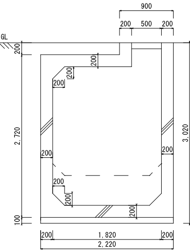
B-B' 断面図 s=1/30
