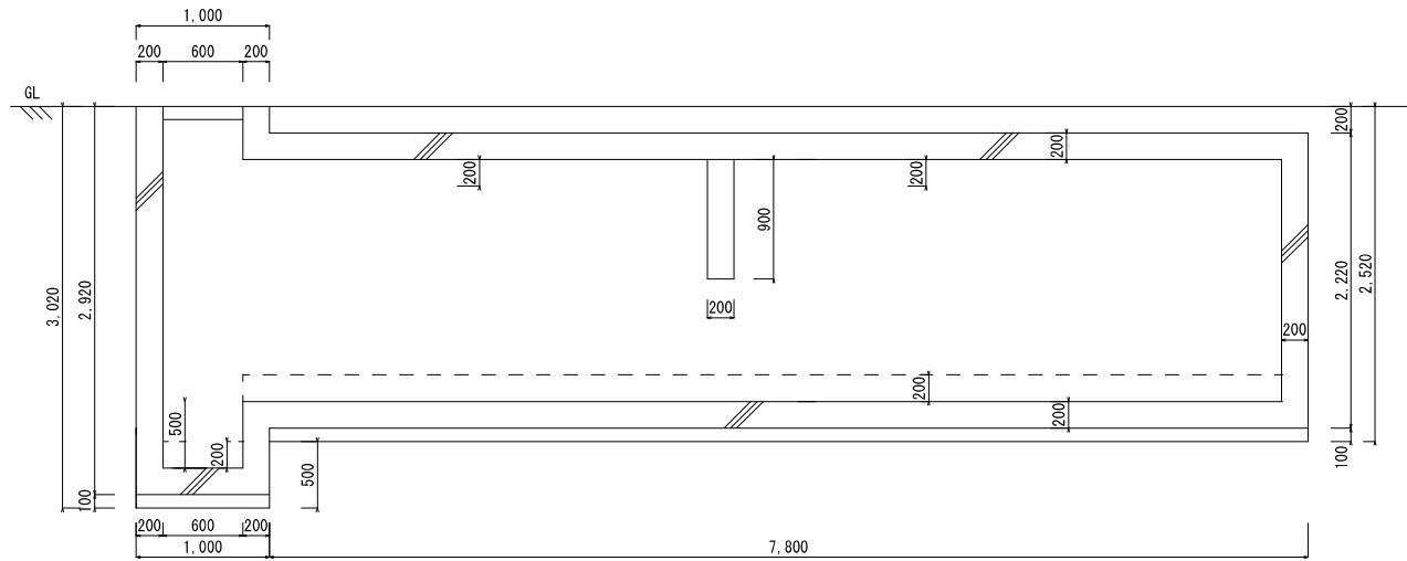
A-A' 断面図 s=1/30
