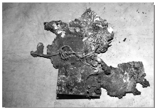
家庭用蓄電池の焼損状況
