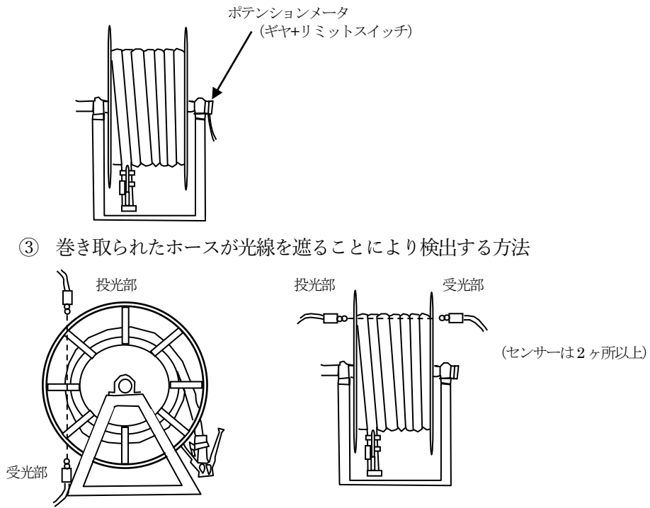
図4-2-1 ホース巻取装置による誤発進を防止する方法
