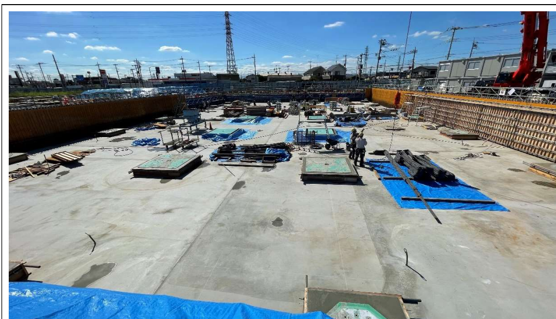
マットスラブ生コン打設の状況 [2024.9月下旬]
