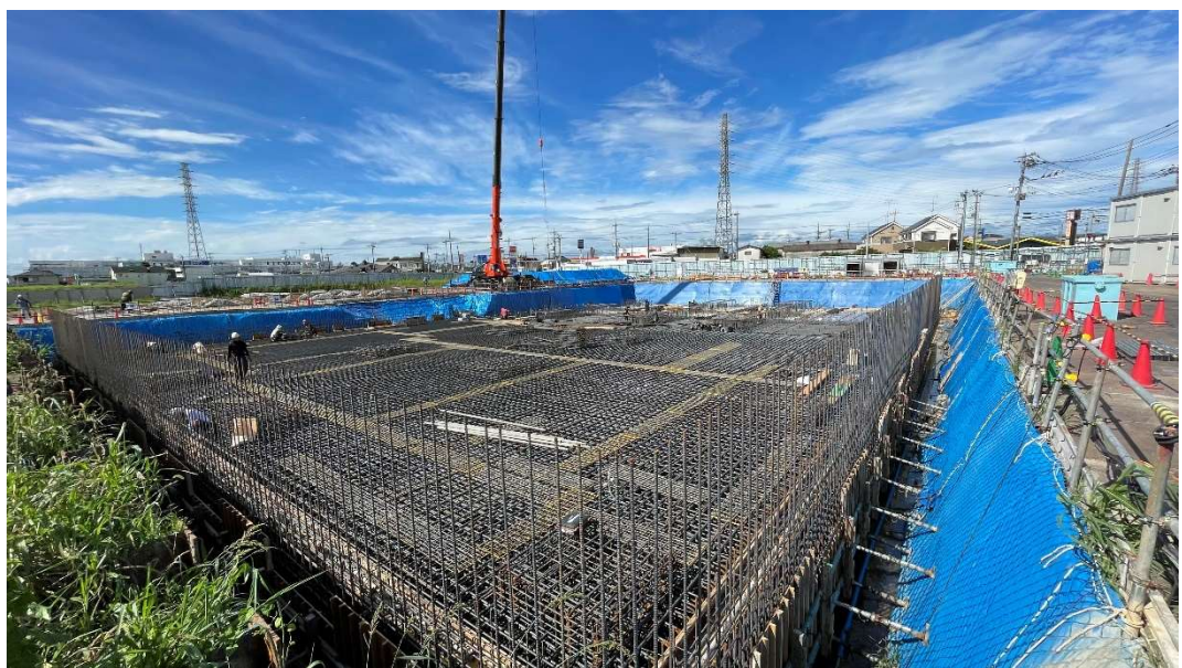
マットスラブ配筋工事の状況 [2024.8月下旬]
