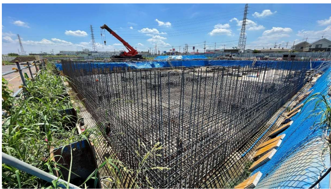
マットスラブ配筋工事の状況 [2024.8月中旬]
