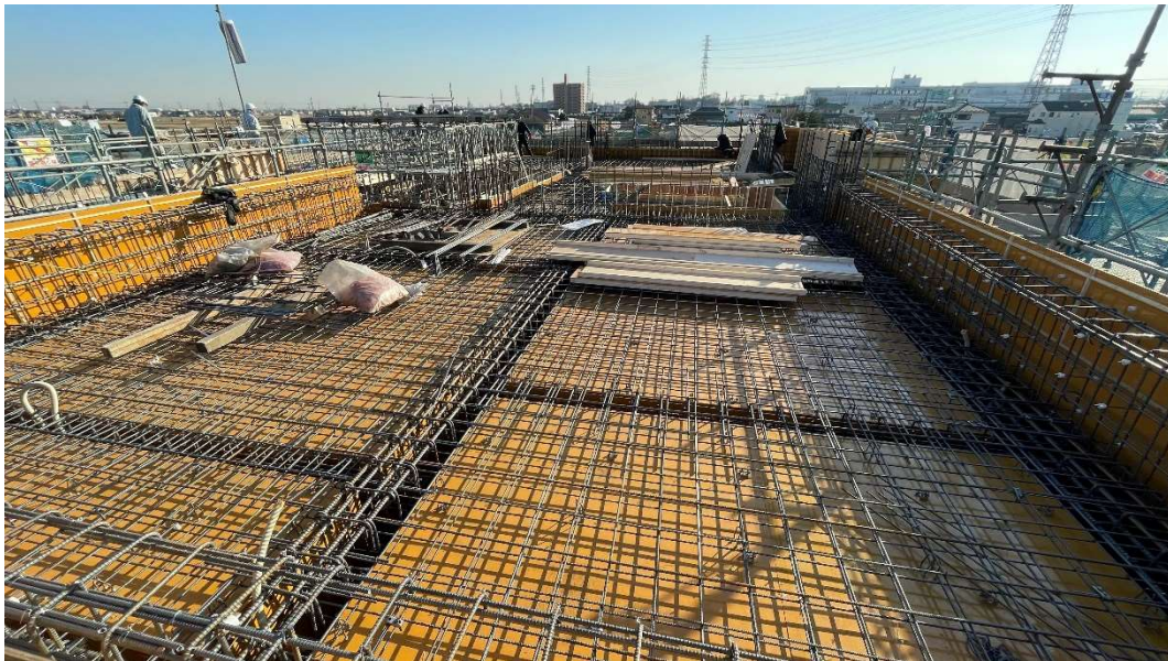
2階床配筋工事状況 [2025.12 月中旬]
